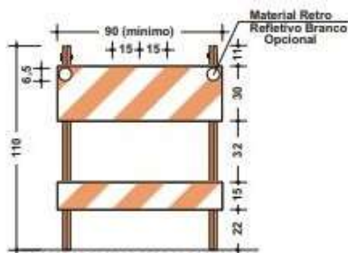
Elevação Frontal medidas em centímetros
