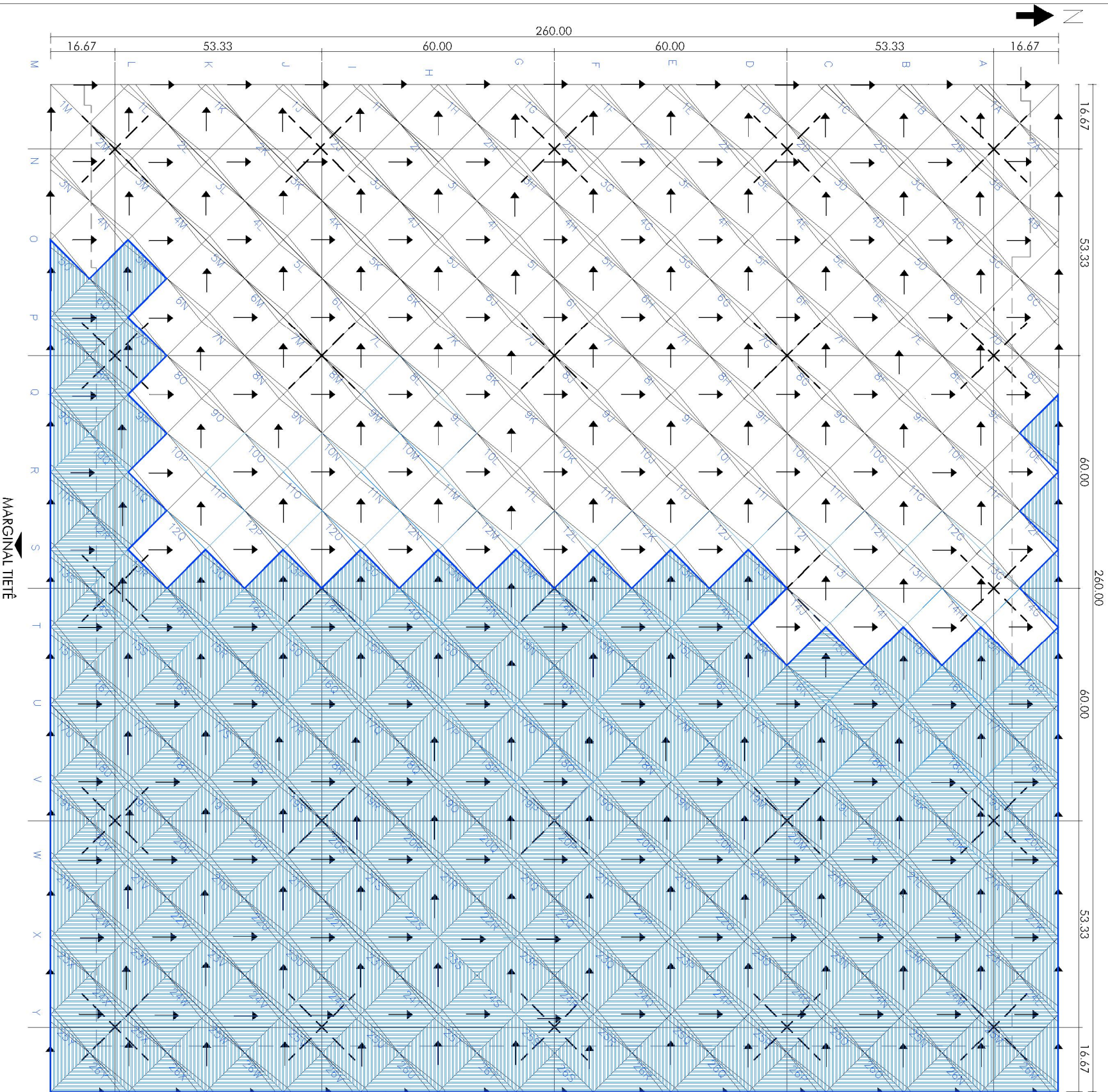
ÁREAS DOS MÓDULOS DO TELHADO - esc. 1:750
