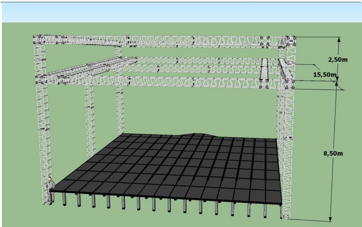
Estrutura base (representação gráfica) – Palco Especial DANÇA
