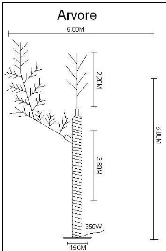
Figura 2 – Dimensões do adorno em forma de árvore
