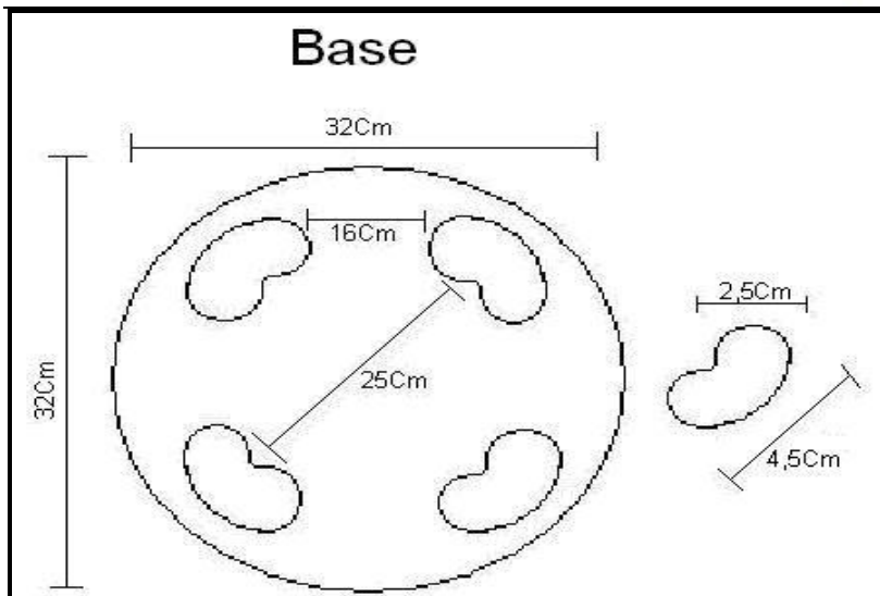
Figura 3 – Dimensões da base de fixação.
